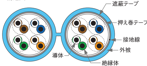
■構造図
