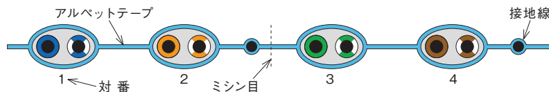
■構造図
