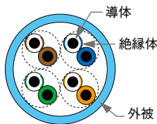
■構造図
