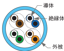
■構造図
