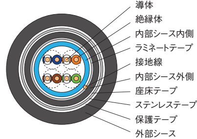
■構造図
