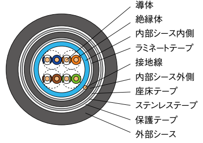
■構造図
