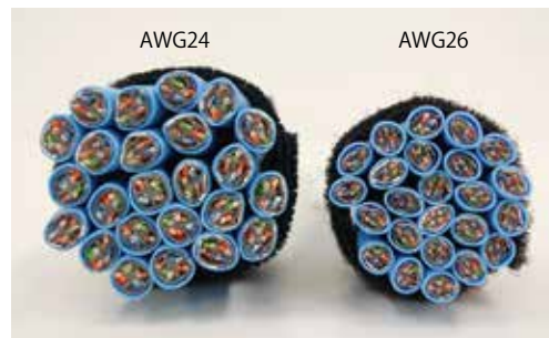
左: 0.5-4P NSGDT6-10G-S 1本辺りの外径7.5mm 右: 26AWG-4P SD-10G-S 1本辺りの外径6.0mm
