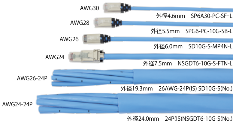
左: 0.5-4P NSGDT6-10G-S 1本辺りの外径7.5mm 右: 26AWG-4P SD-10G-S 1本辺りの外径6.0mm
