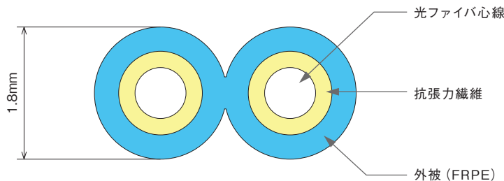
■構造図
